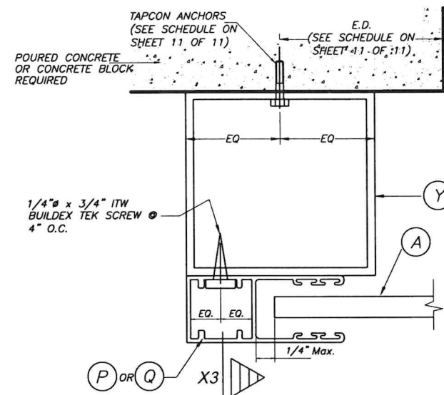
SECTION P - P (3) : BUILD-OUT N.T.S.
