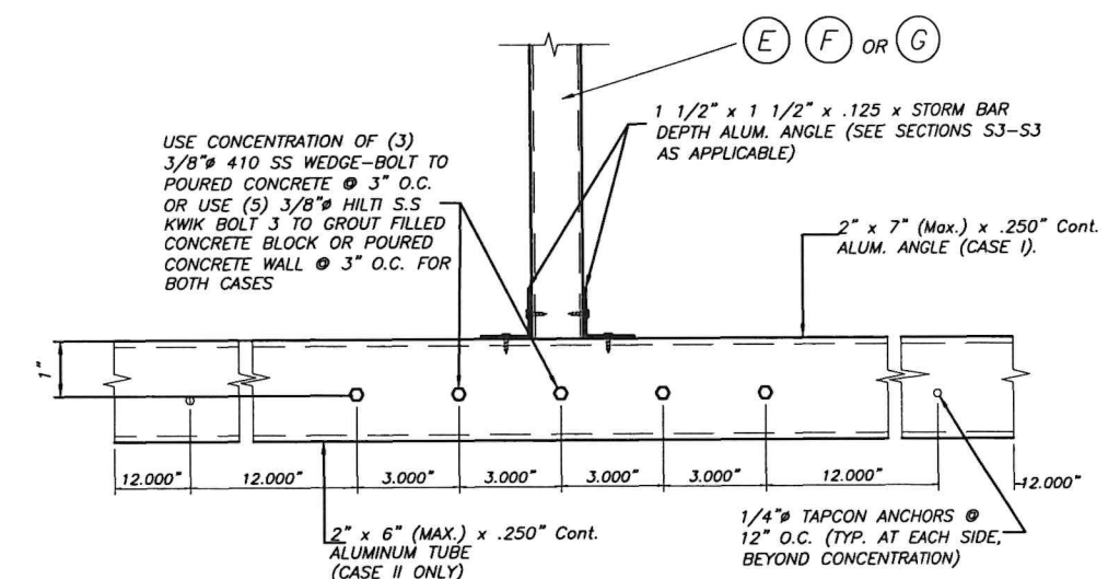
ELEVATION X SCALE : N.T.S.
