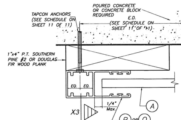
SECTION P - P (3) : B.O. (OPTION) N.T.S.
