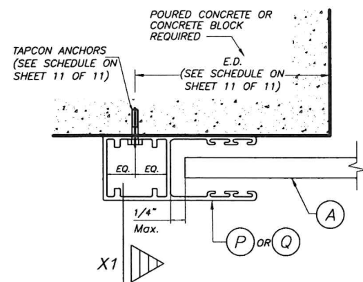
SECTION P - P (1) : WALL MOUNT N.T.S.
